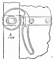
Fig. 2759. Simms Lock.
